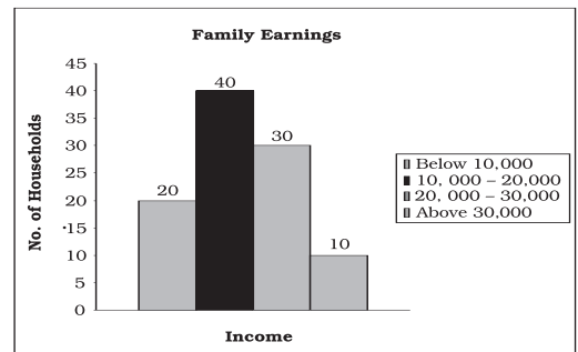
Fig. 8.3: Histogram
